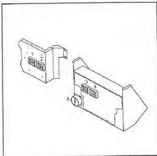
Fig.1a. A=hoofdschakelaar
